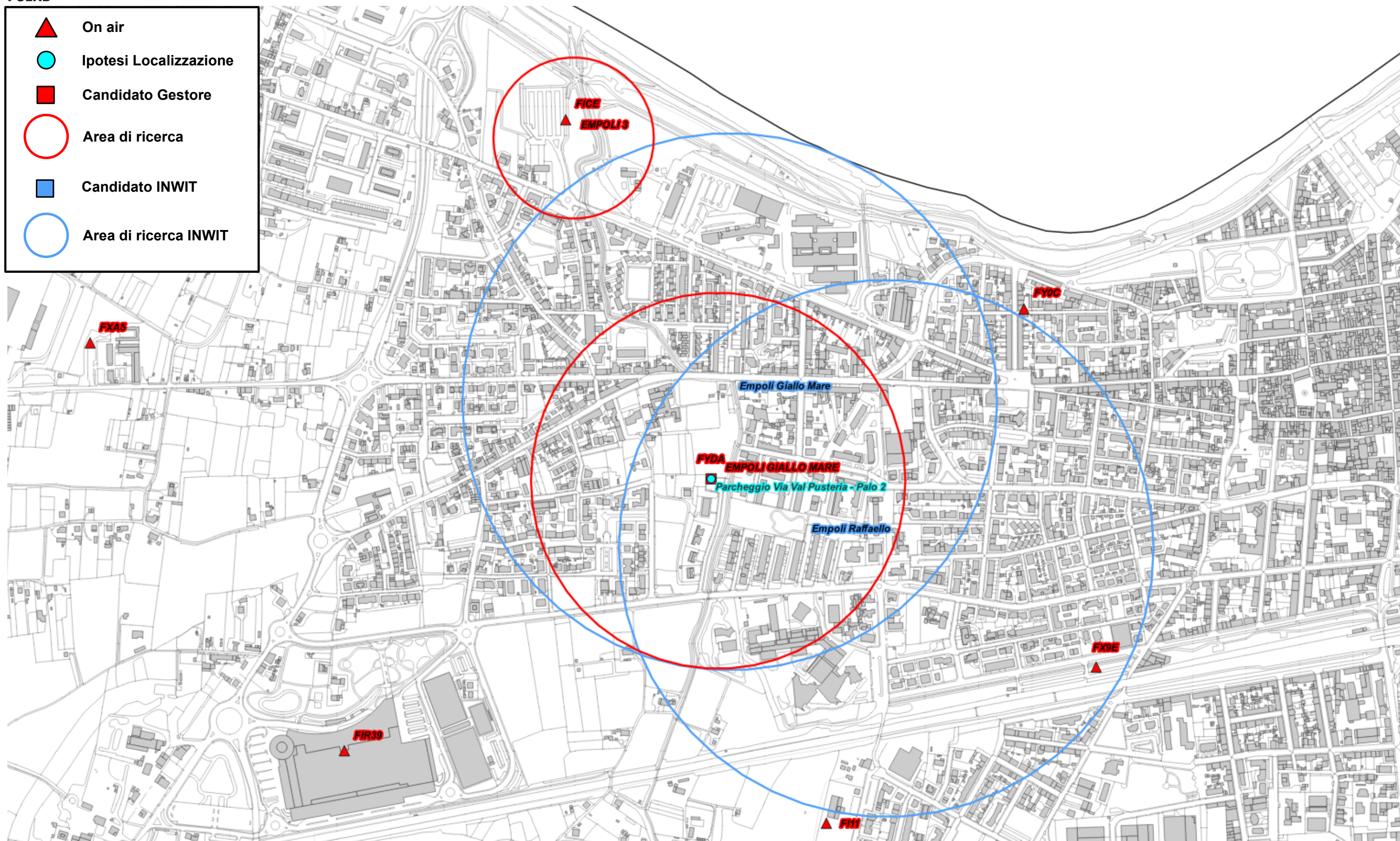
Fig. 26 Dettaglio piano di rete - Gestore TIM
