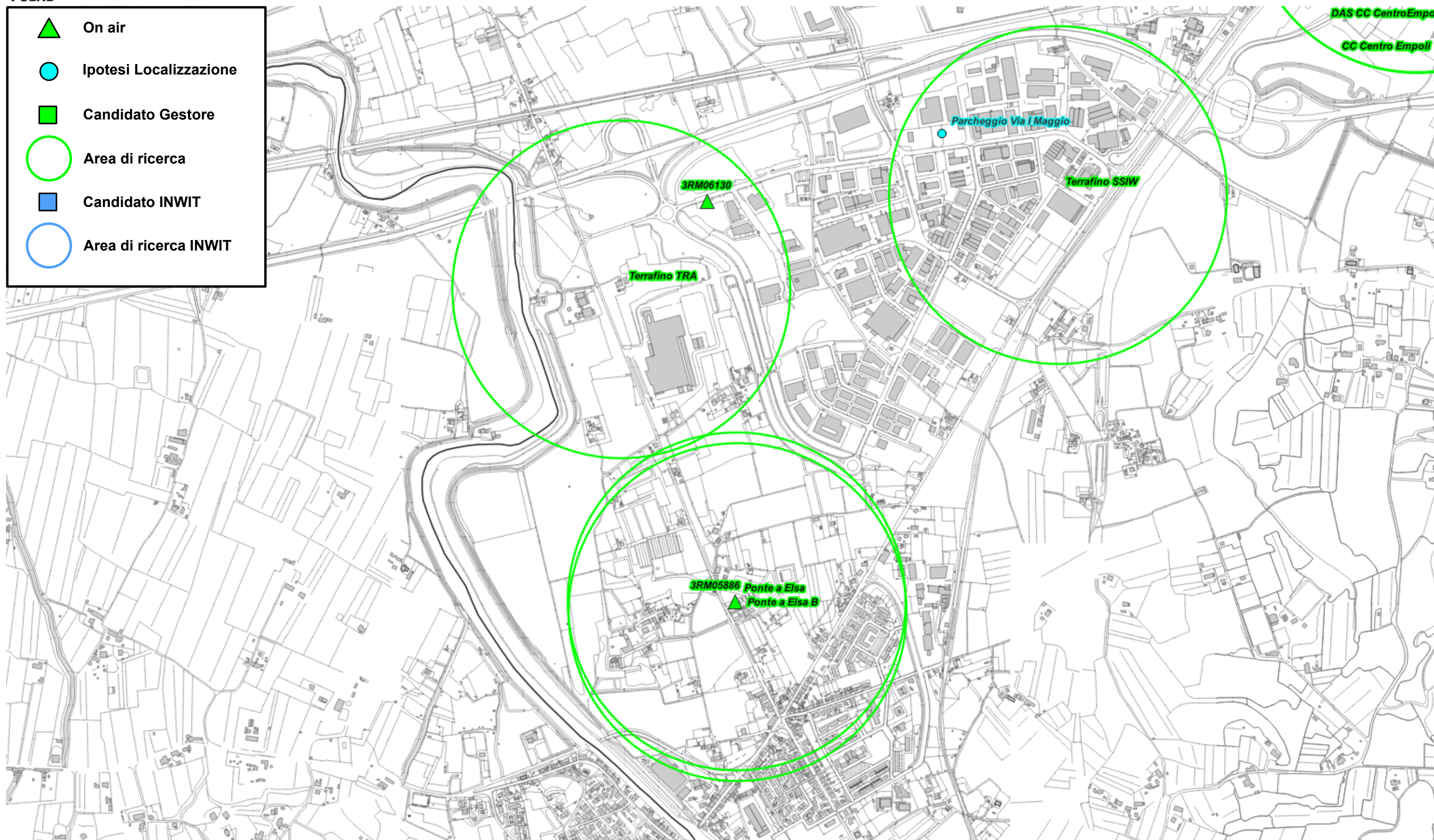
Fig. 34 Dettaglio piano di rete - Gestore VODAFONE
