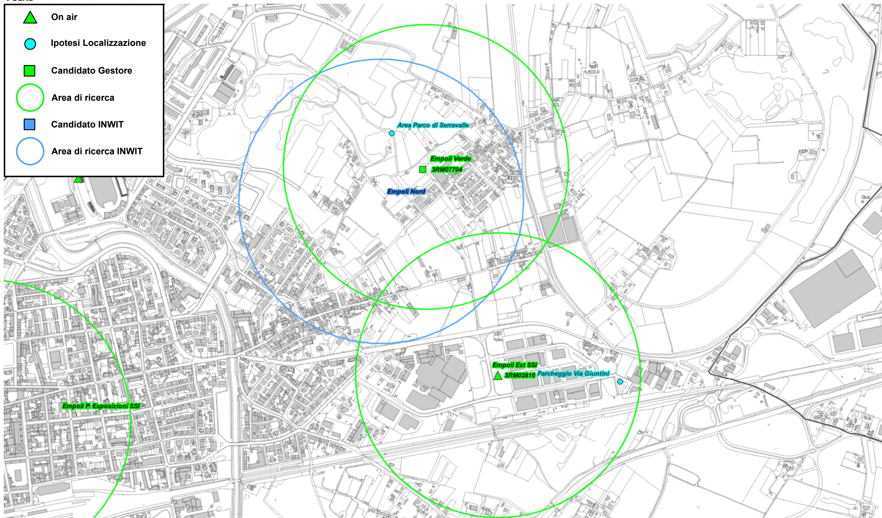
Fig. 33 Dettaglio piano di rete - Gestore VODAFONE
