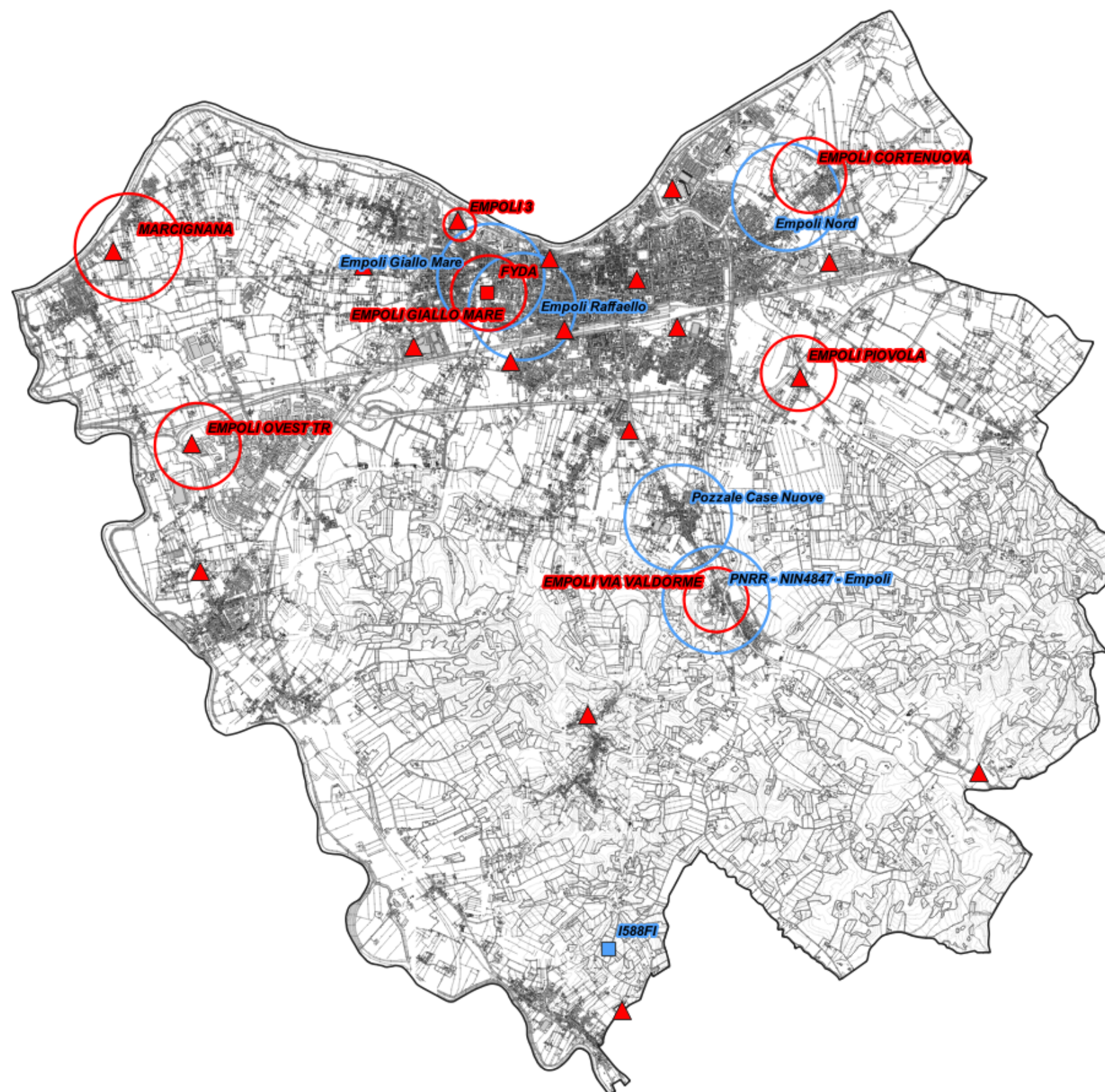
Fig. 23 Piano di rete - Gestore TIM
