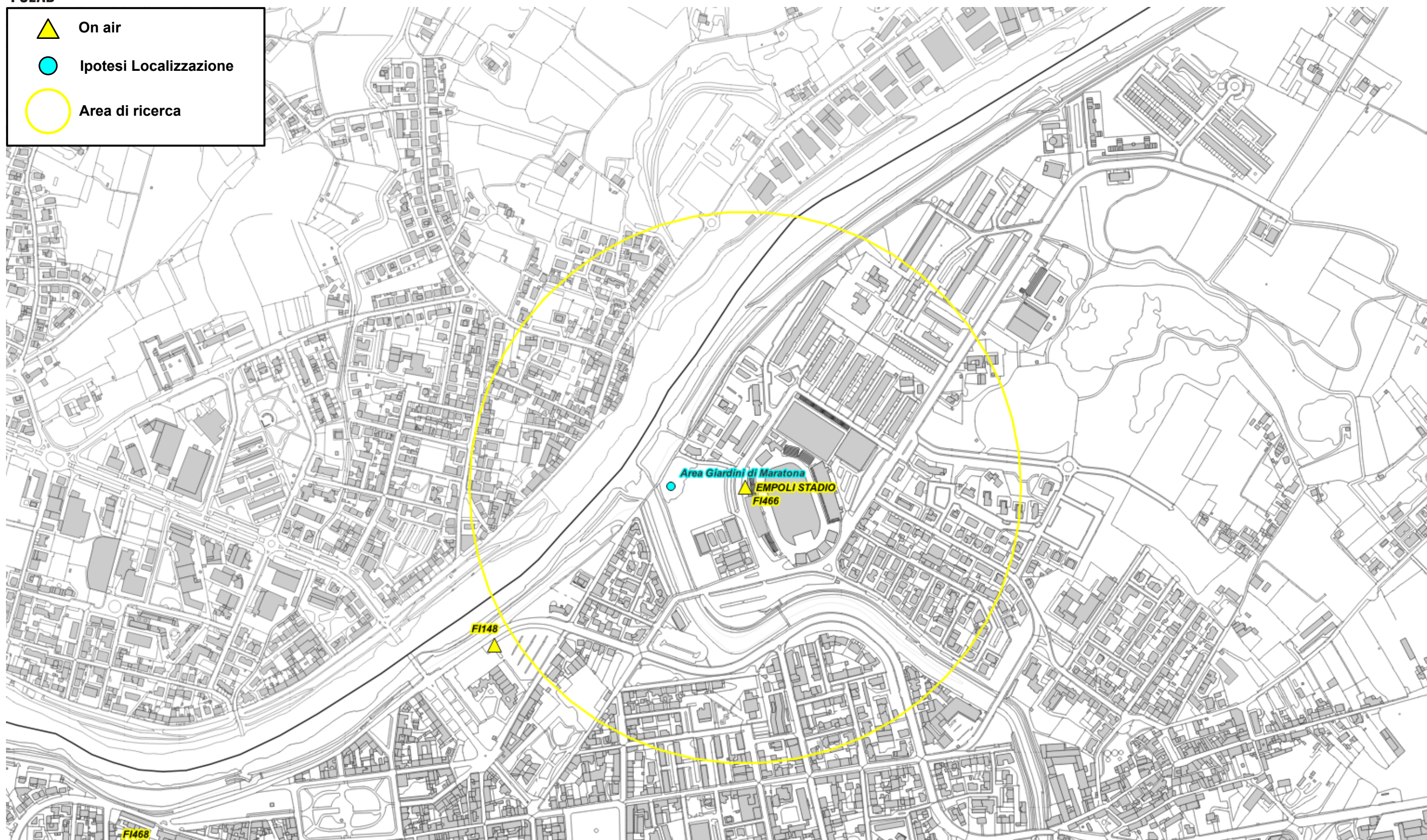
Fig. 38 Dettaglio piano di rete - Gestore WINDTRE
