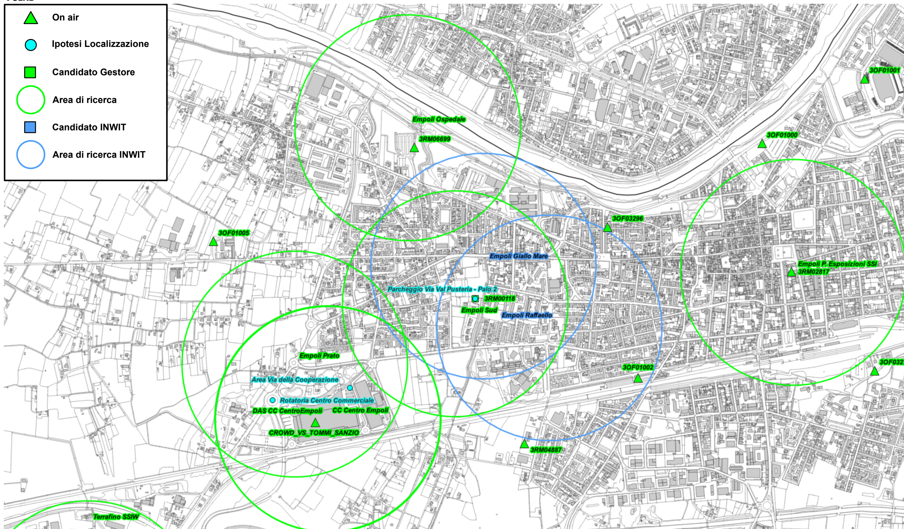
Fig. 32 Dettaglio piano di rete - Gestore VODAFONE
