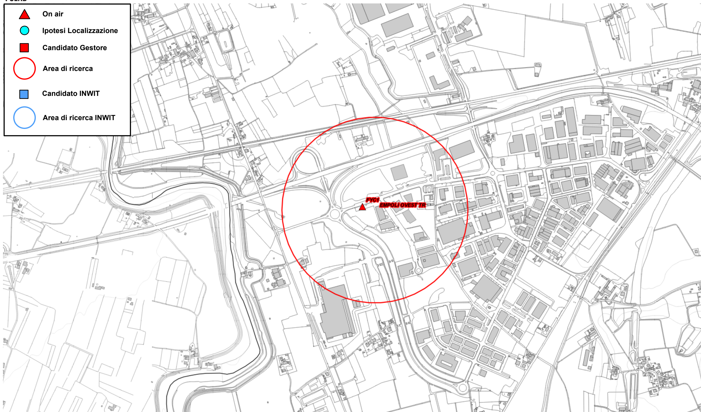
Fig. 25 Dettaglio piano di rete - Gestore TIM
