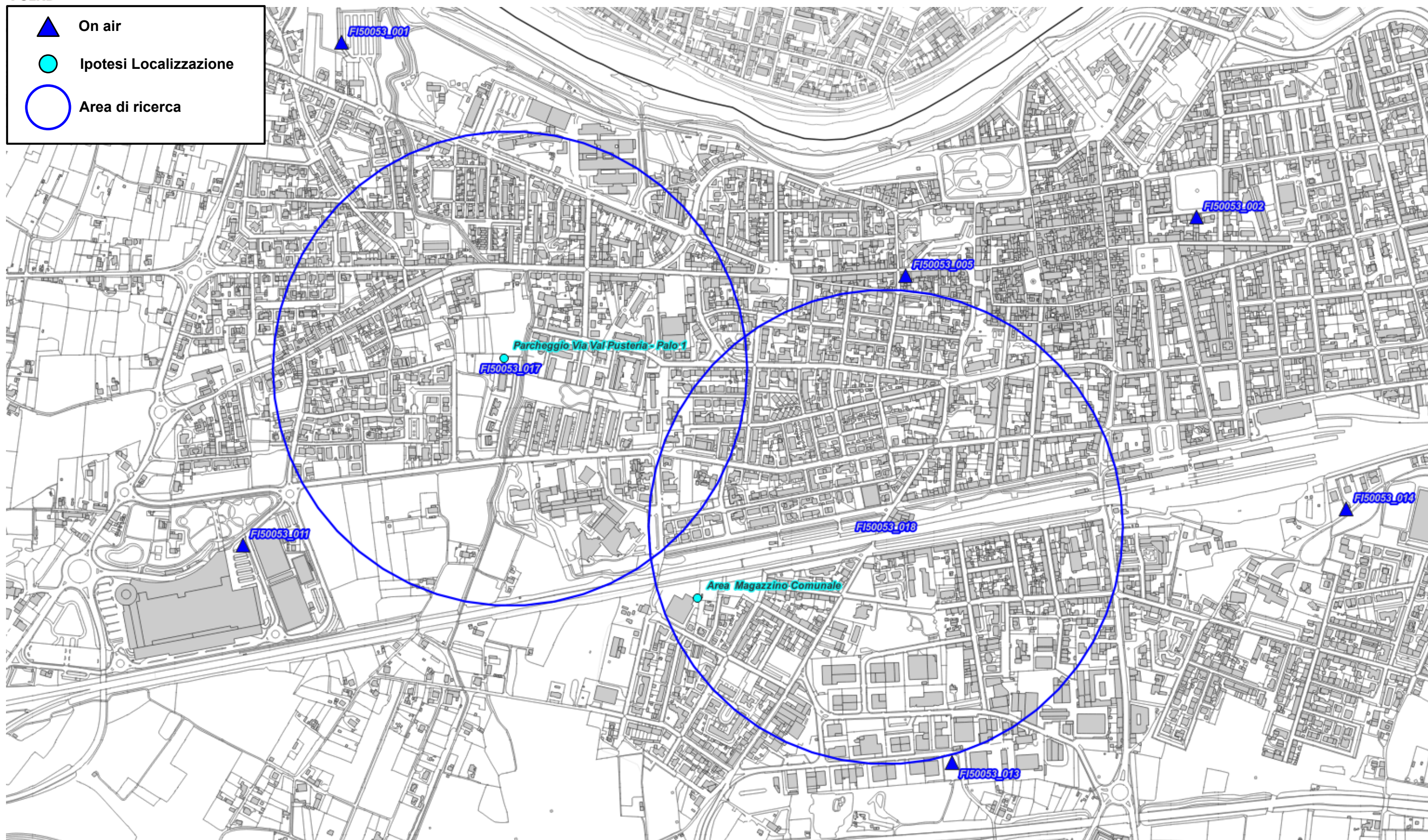
Fig. 41 Dettaglio piano di rete - Gestore ILIAD
